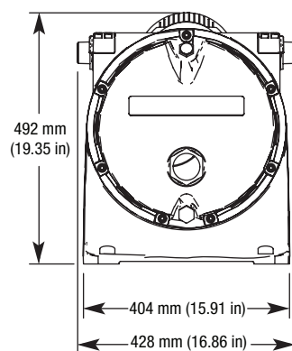
Bombas peristálticas EP4
