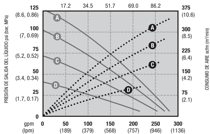
Rendimiento de la bomba Husky 3300
