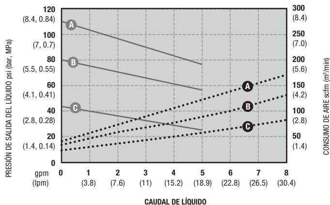
Rendimiento de la Fast-Flo 1:1
