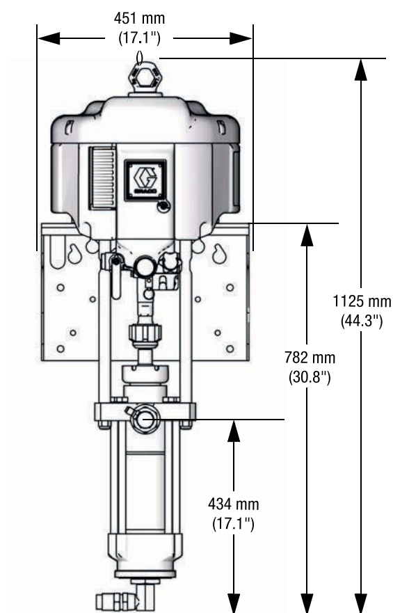
Conjunto de montaje en pared 247550
