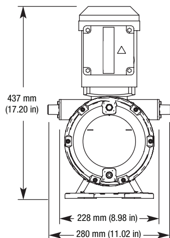
Bombas peristálticas EP2
