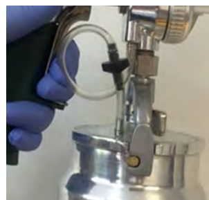
Válvula anti-retorno
